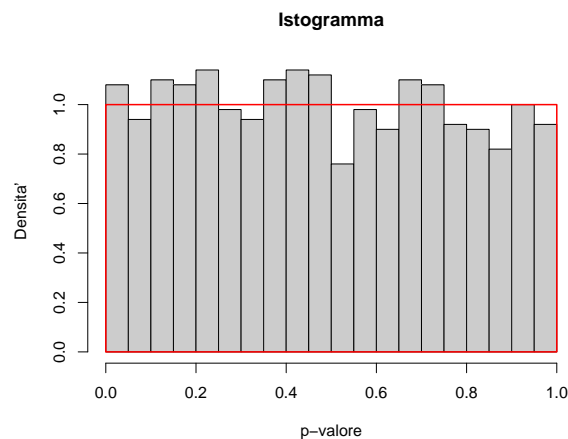
Figura 8: Istogramma p-valore
